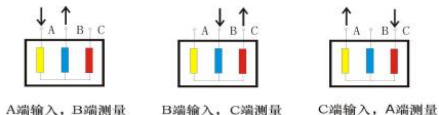
图 4 Y 接线
