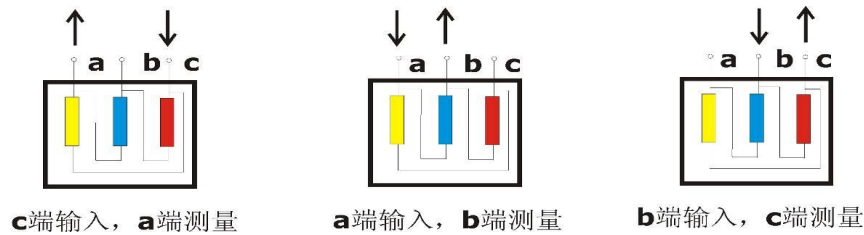
图 5 内连接 \Delta 接线
