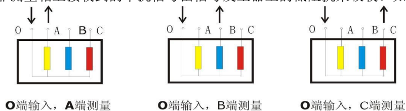
图 3 YN 接线
